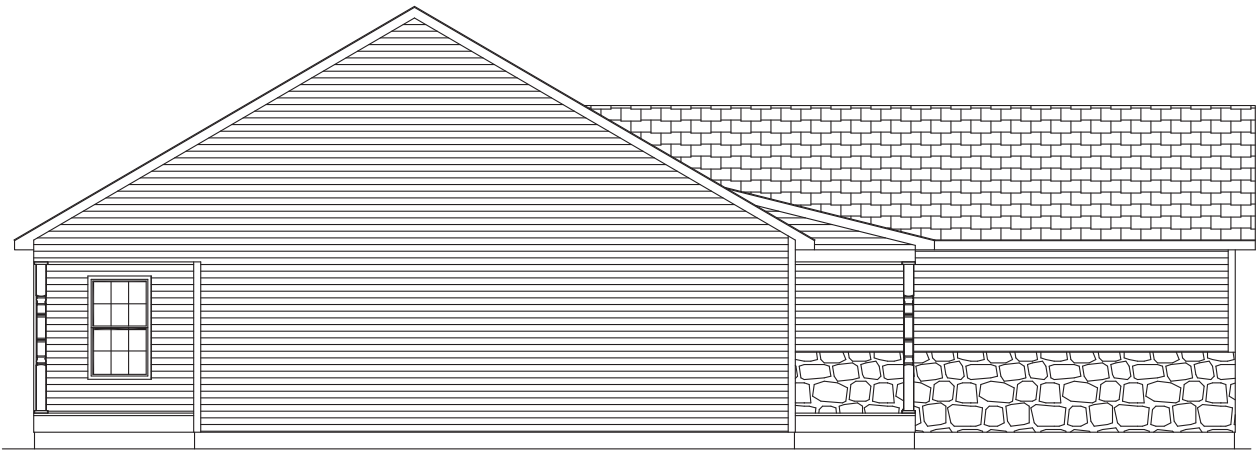
RIGHT ELEVATION
